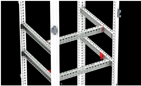
Atkı üzerinde genişlik bağlantısı (dikey pozisyon)
