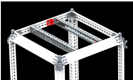
Gövde üzerinde üst bağlantı (dikey pozisyon)
