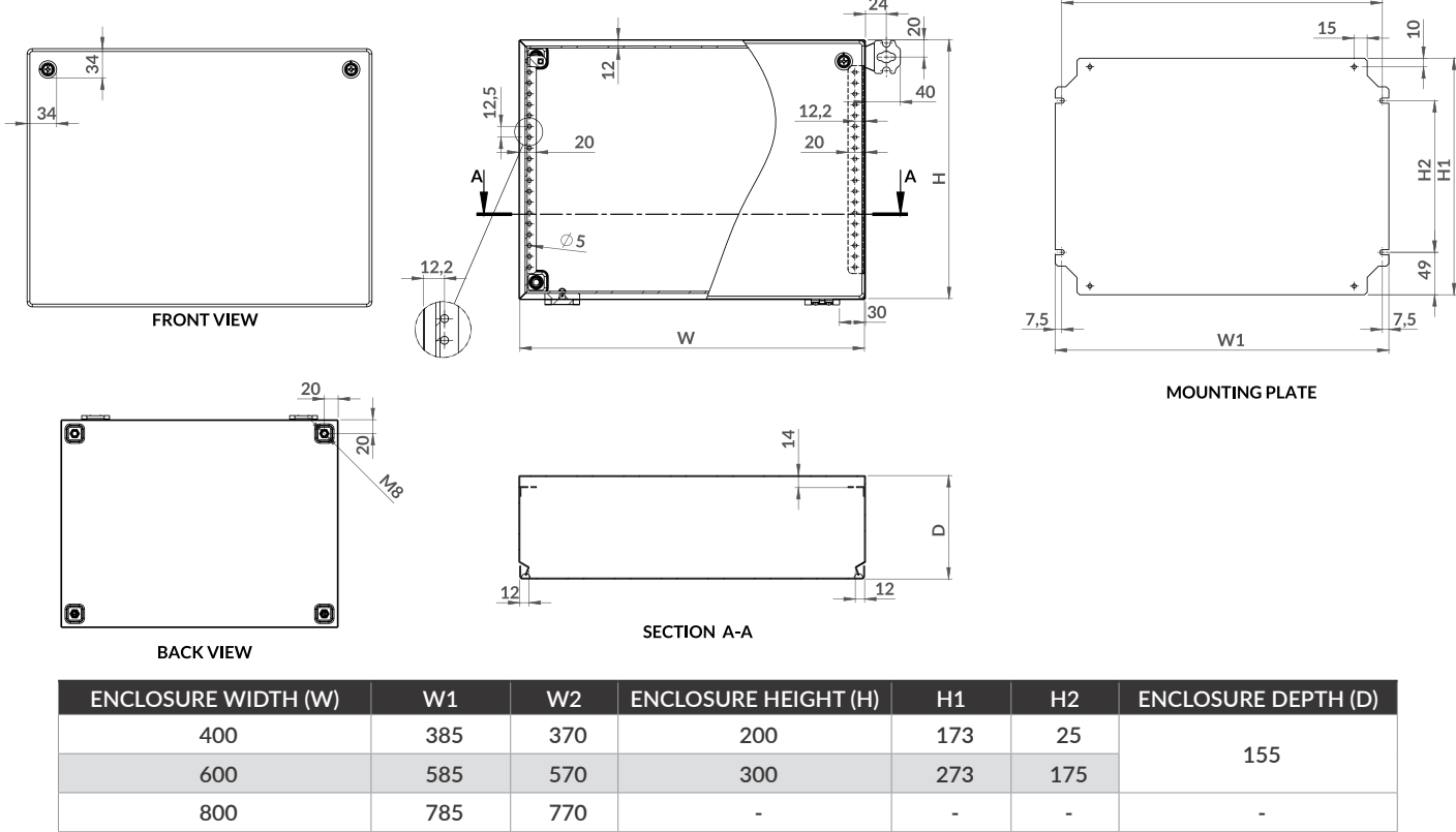
KT SOLID DOOR BUS BOX
